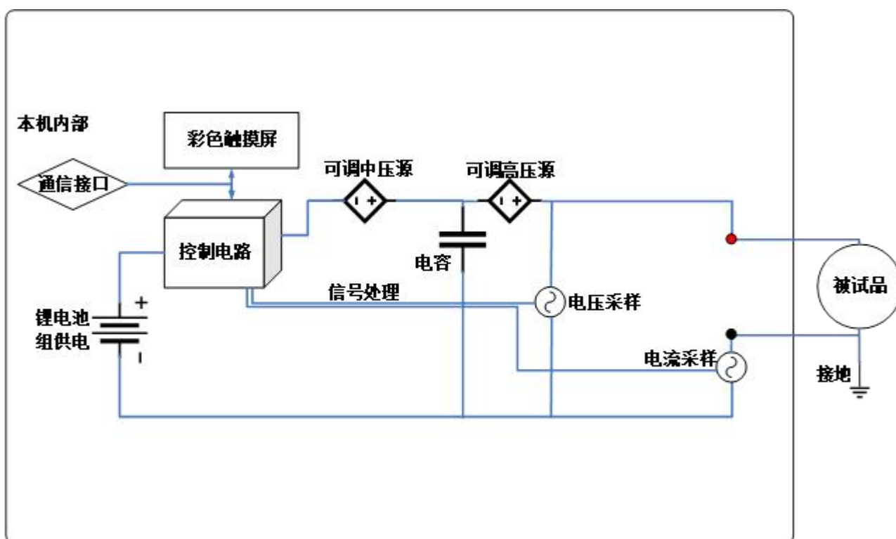
图 2 测试原理图
