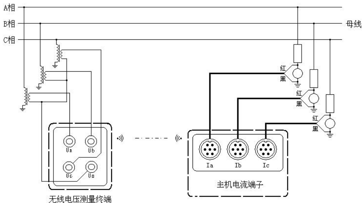
图十六、无线测试接线图
