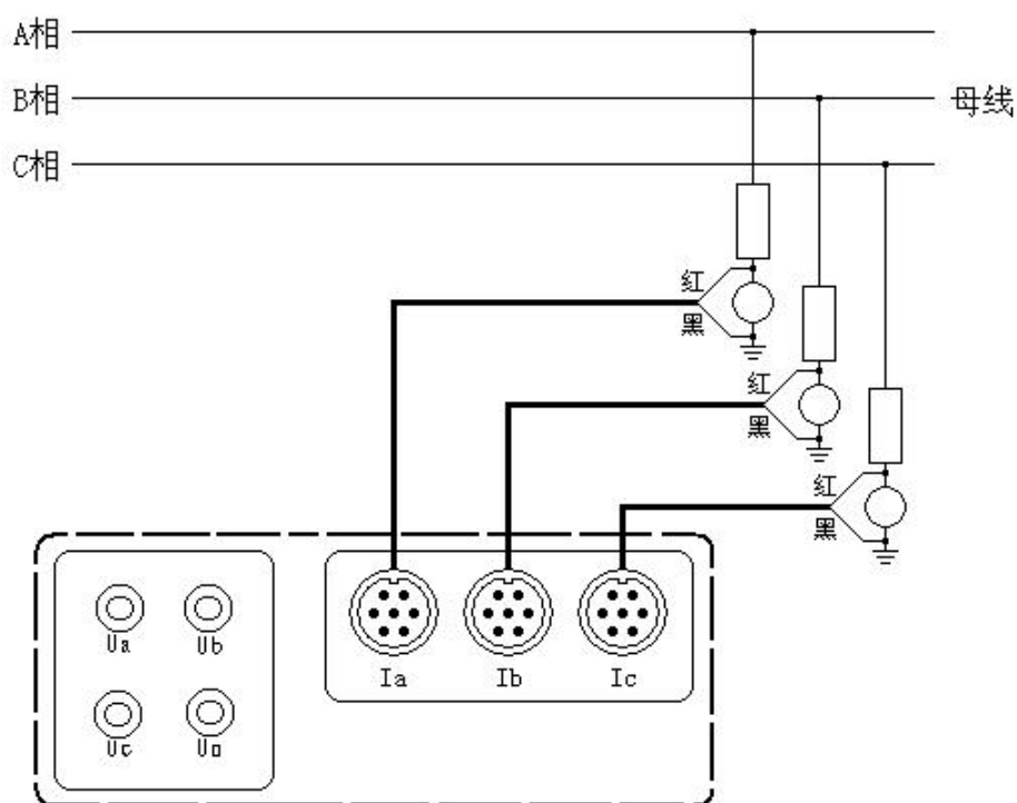
图十七、无 PT 测试接线图
