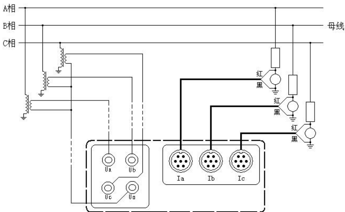
图十五、有 PT 测试接线图
