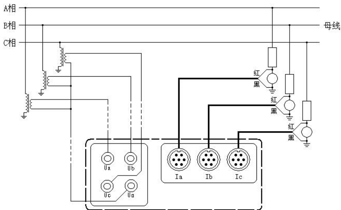
图十四、有 PT 测试接线图
