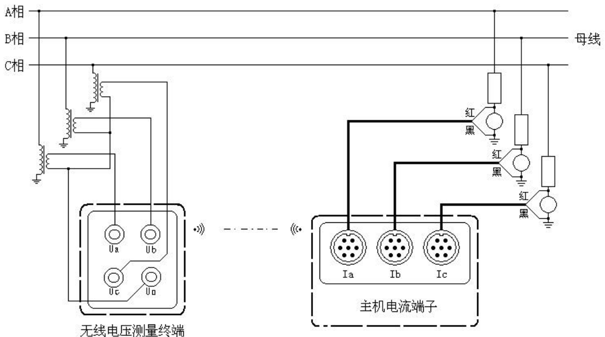
图十五、无线测试接线图
