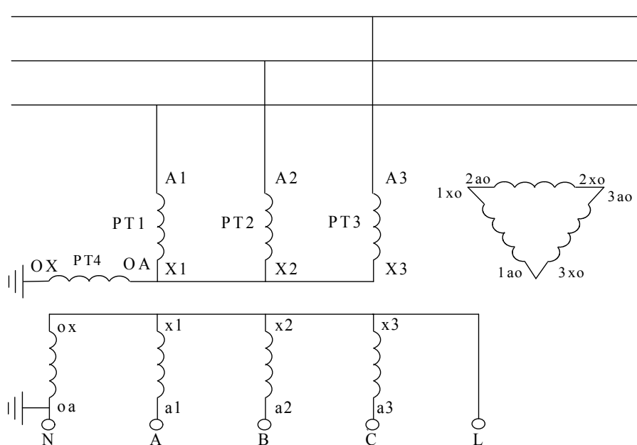
图 8 4PT 连接方式 1
