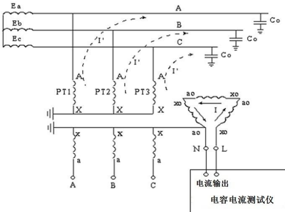
图 1 测量原理图
